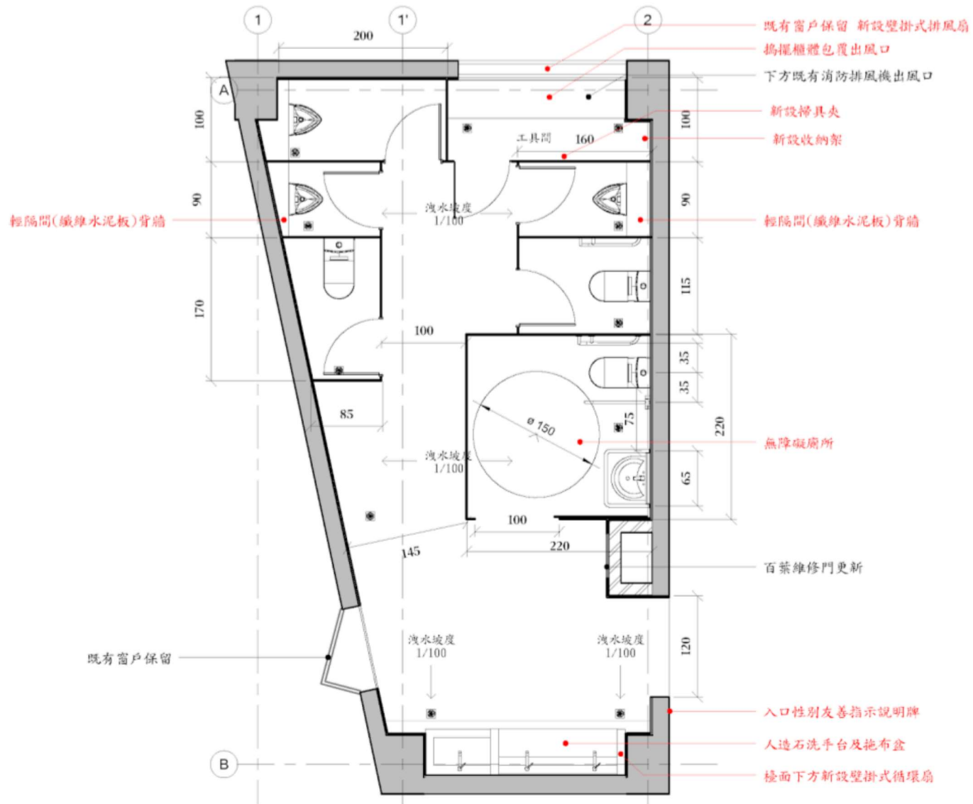
性別友善廁所平面圖
